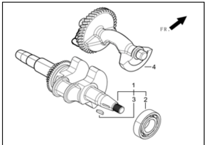
Fig. 4 - Crankshaft
