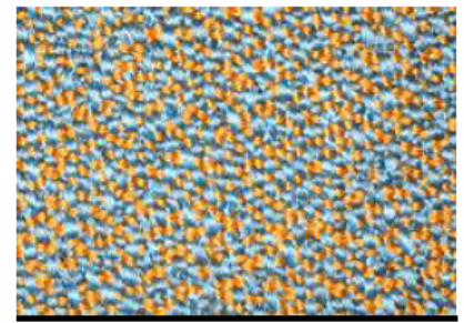
SERA mirage
