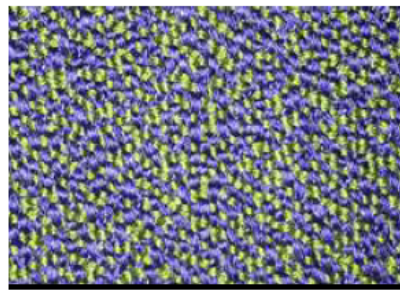
SERA mare
