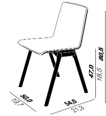
F2S-PP
