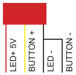
BUTTON WIRING
