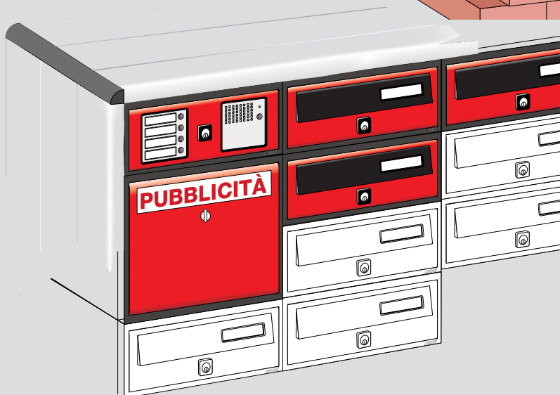
Composizione con mantello, sportello SP1 270 ACC predisposto per l'inserimento di campanelli, telecamera, citofono e numero civico per i modelli Bticino Sfera e corpo doppio pubblicità. Accessori vedi da pag. 71.
