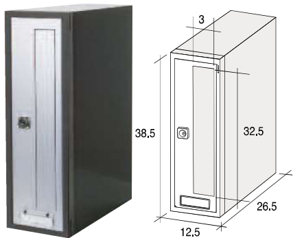
Esempio cassetta Modular 1V: Corpo (C1) + Sportello (SP1V)
