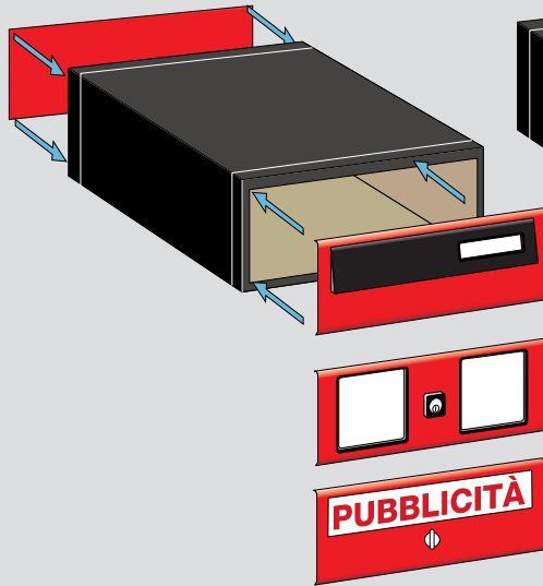
Composizione con mantello da recinzione Configuration with outer casing for fence mounting
