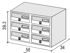
JUMBO 6 Blocchiera da 6 cassette 6 unit mailbox set
