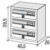
JUMBO 3 Blocchiera da 3 cassette 3 unit mailbox set
