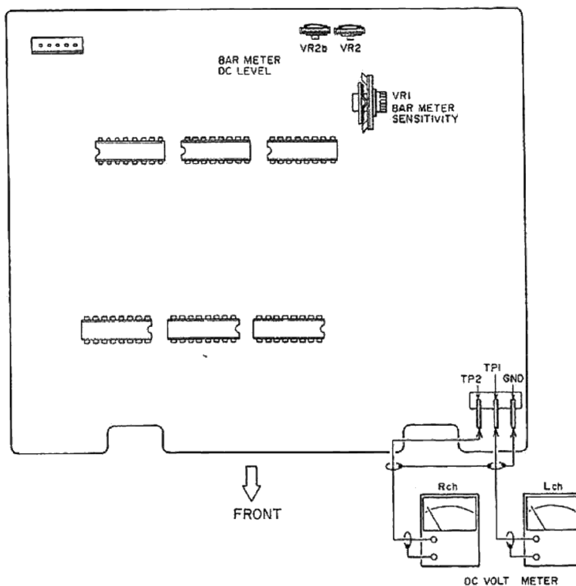
Fig. 46 Bar Meter P.C Board T1009A5020
