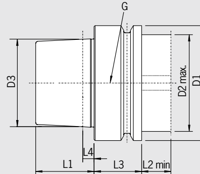
HSK-E
