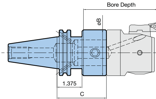
DIN B Coolant Holes
