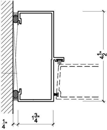
1. Door Jamb Detail
