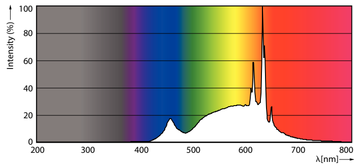
75W E26 A21 930 Frosted
