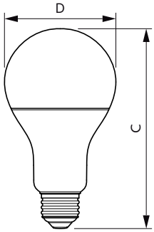
A21 120V 12.2-75W 1100lm 3000K E26 D
