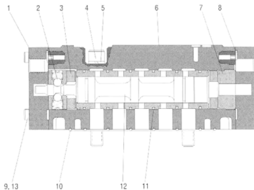
TB-1510 Spool Valve
