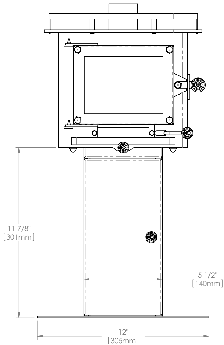
POÊLE MINI CUBIC CB-1008 SUR PIEDESTAL CB-2014 CUBIC MINI STOVE CB-1008 ON PEDESTAL CB-2014
