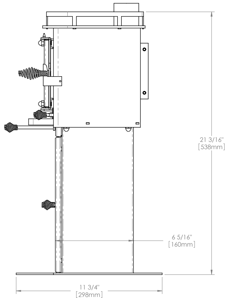
POÊLE MINI CUBIC CB-1008 SUR PIEDESTAL CB-2014 CUBIC MINI STOVE CB-1008 ON PEDESTAL CB-2014
