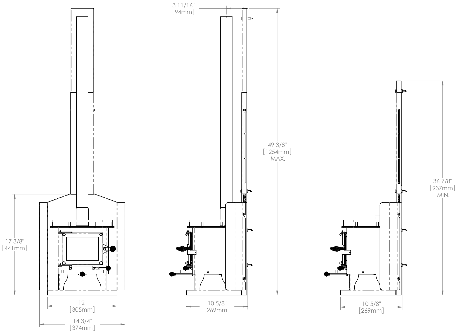
POÊLE MINI CUBIC CB-1008 AVEC FIXATION MURALE CB-2012-SS CUBIC MINI STOVE CB-1008 WITH WALL MOUNT CB-2012-SS
