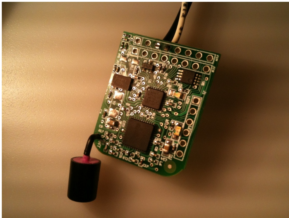
ZT-50 Mini with external antenna (0 dBi)
