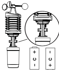
Wind Sensor LTV-W1
